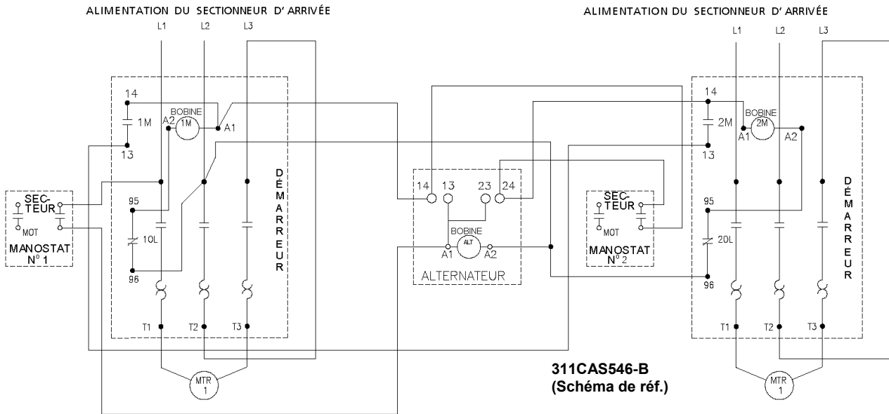
MONOPHASÉ - DÉMARREURS MAGNÉTIQUES DUPLEX A/ ALTERNATEUR
