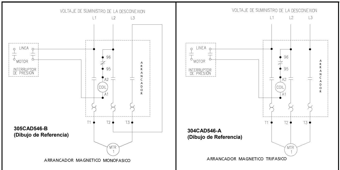
Figura 1-1 Diagrama de Cableado
