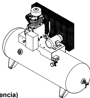
C284-A (Dibujo de Referencia)
