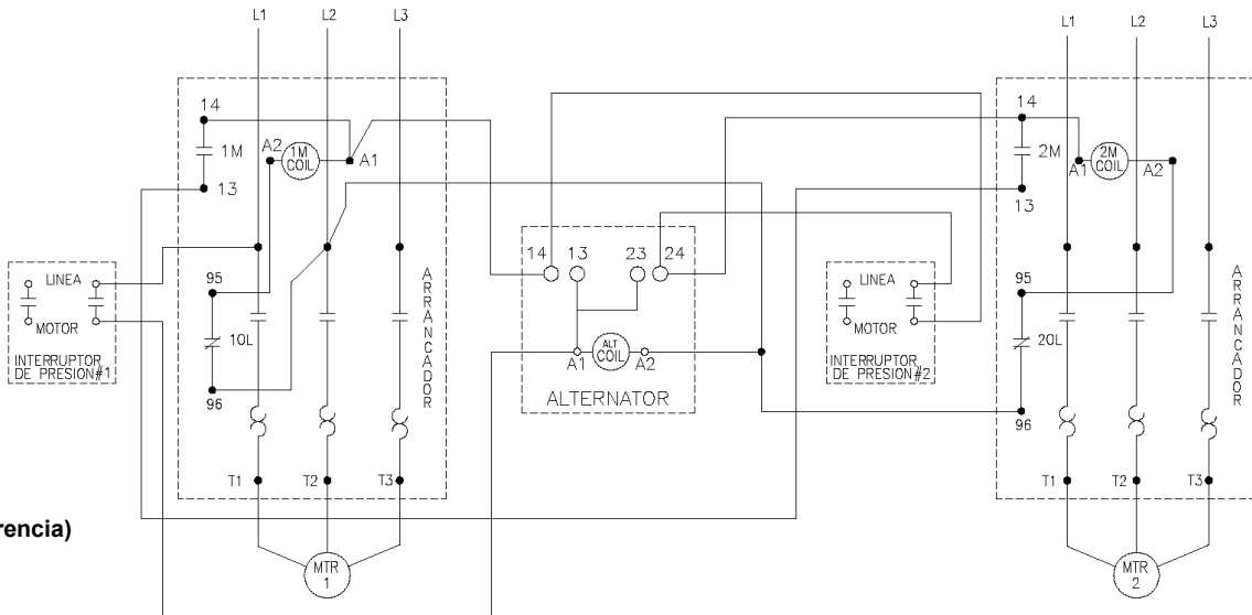
Figura 1-2 Diagrama de Cableado
