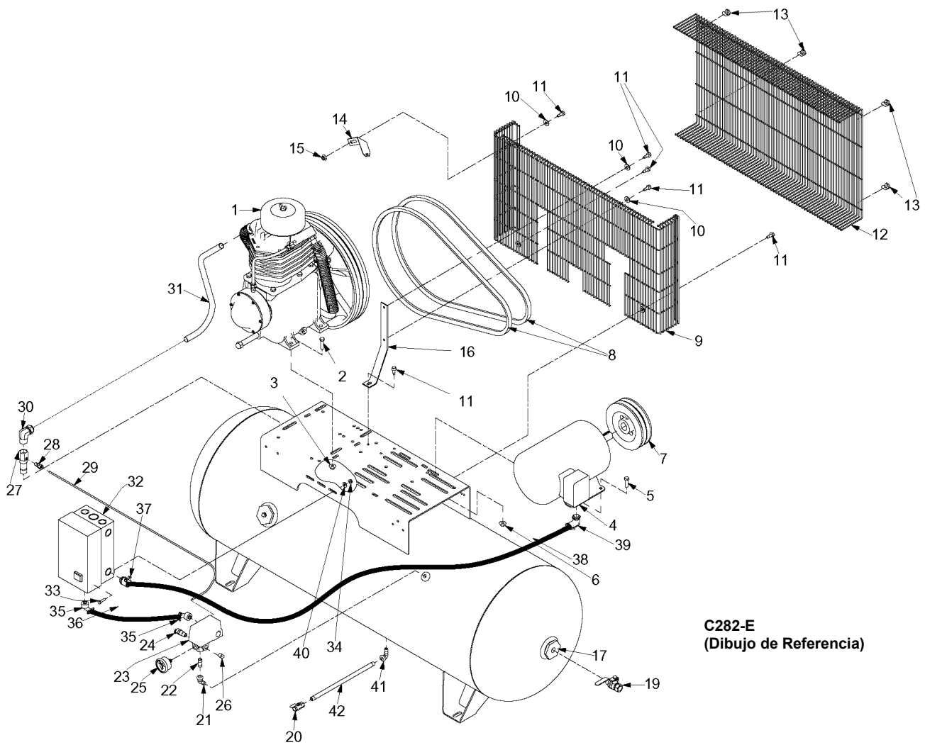
ILUSTRACION DE LAS PARTES DE REPARACION Modelos: 1WD54, 1WD57, 1WD64, 1WD65, 13G708, 13G709
