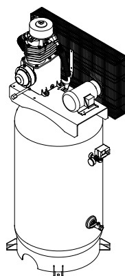
C283-B (Schéma de réf.)
