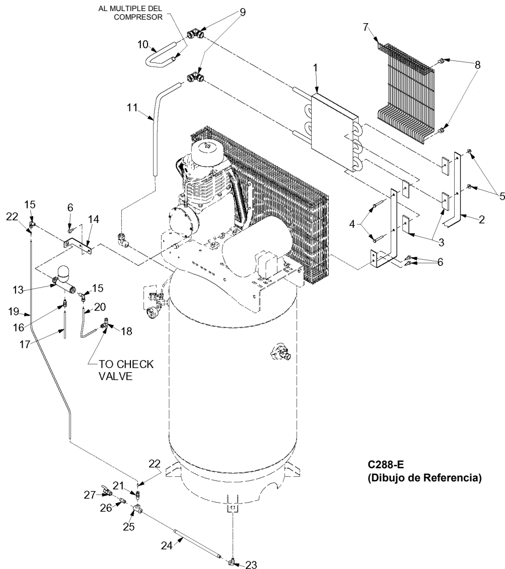
ILUSTRACION DE LAS PARTES DE REPARACION Modelos: 4XA61, 4XA62, 1WD58, 1WD63, 13G706, 13G707
