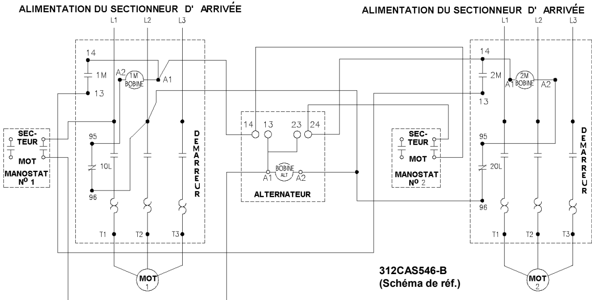
TRIPHASÉ - DÉMARREURS MAGNÉTIQUES DUPLEX A/ ALTERNATEUR
